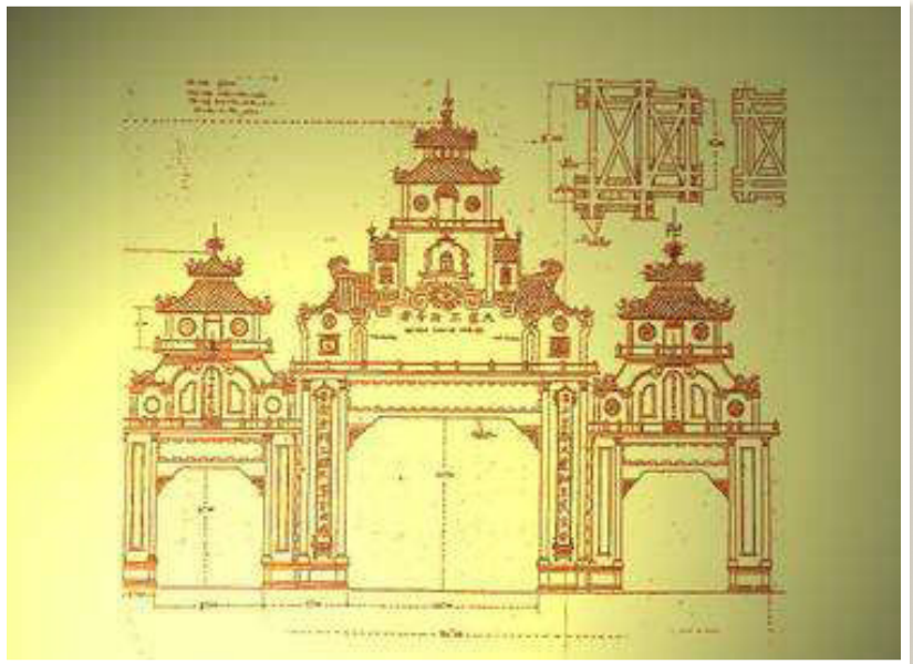
Họa đồ Chánh môn của Ban Kiến Trúc vẽ theo lệnh của Đức Phạm Hộ Pháp
